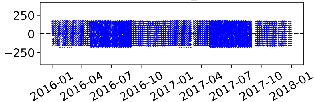
(d) SubStar_Lon
