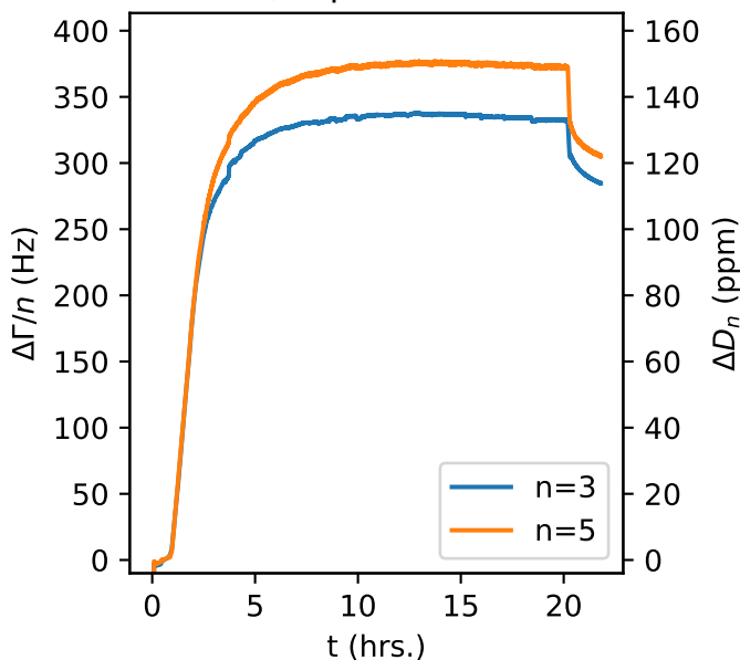
D) non-equilibrated
