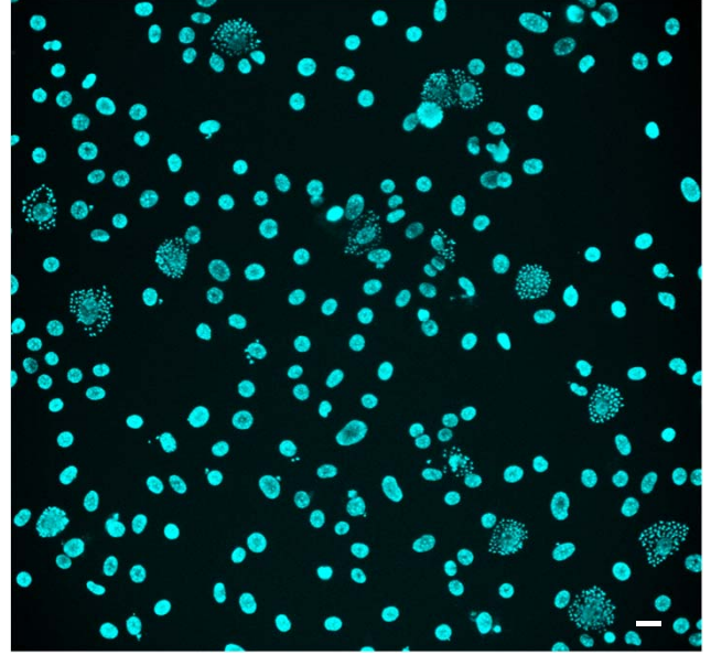
TcPAR1 -KO
