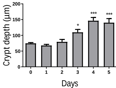
Jejunum
