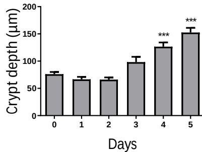
Ileum
