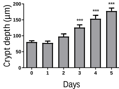
Duodenum
